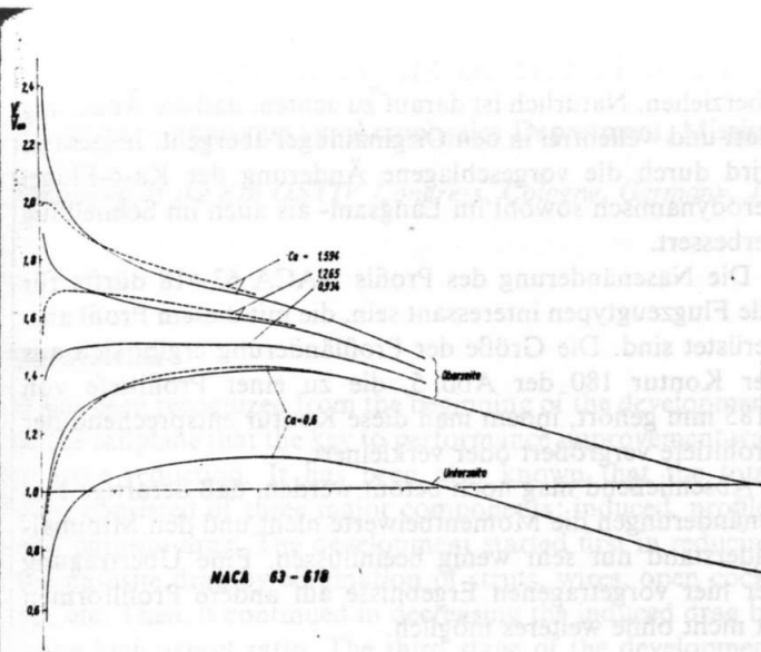
Abb. 4 Geschwindigkeitsverteilung des Profils NACA 63-618 für verschiedene Auftriebswerte. Gestrichelt: erwünschte Variation der Geschwindigkeitsverteilung.
