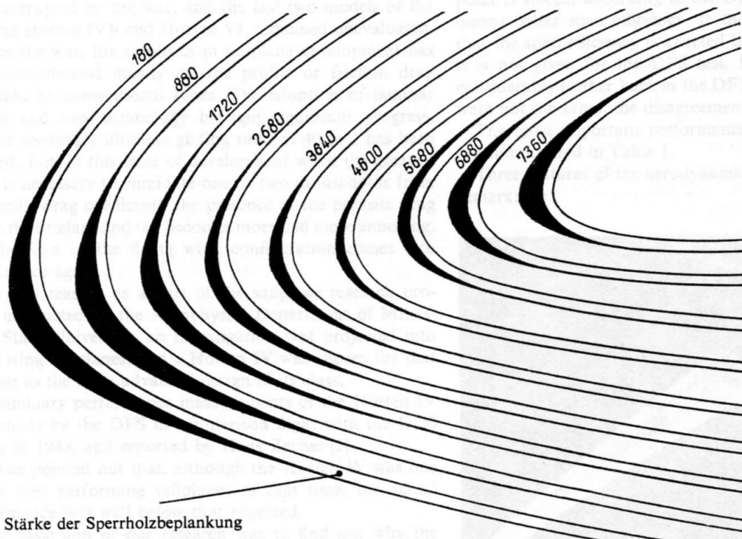
Abb. 5 Straakplan der Flügelnase des Segelflugzeuges Ka 6. Die Ziffern geben den Abstand der Profile von der Mittellinie des Gesamtflügels an. Die schwarz gezeichneten Bereiche sind die vorgeschlagenen Änderungen der Profile; vgl. Abb. 1 und 3.
